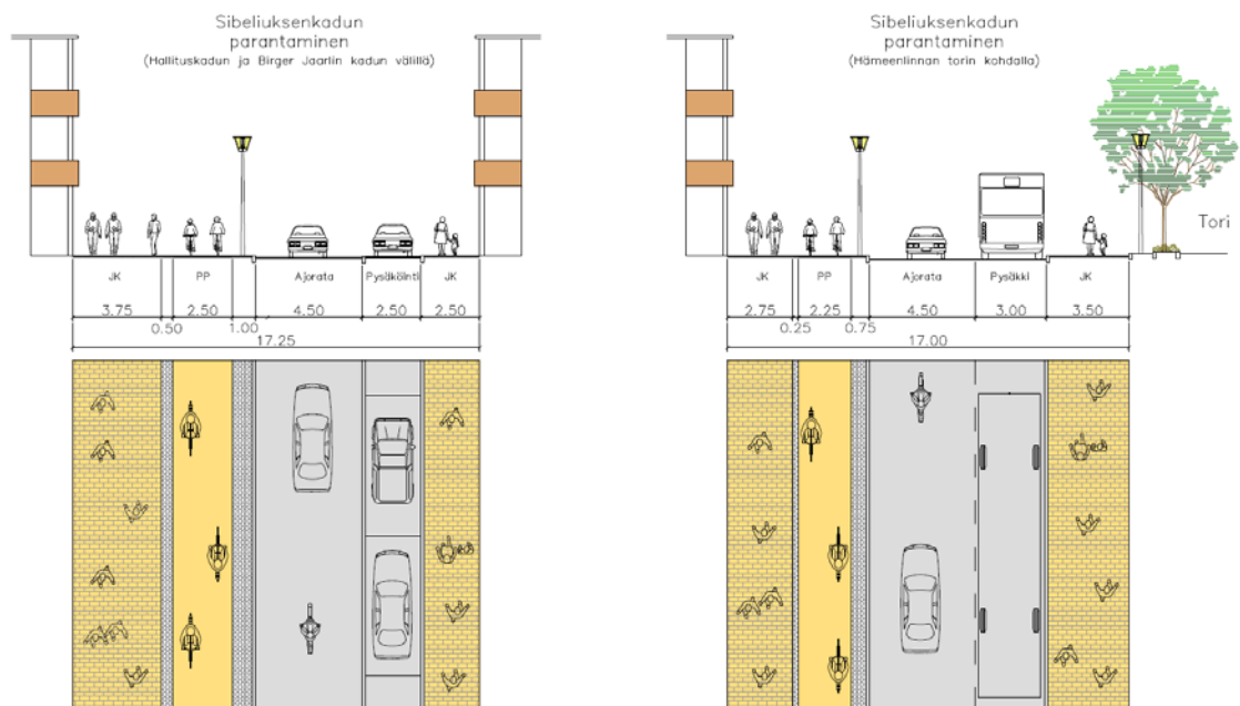
Kuva 17. VE A Sibeliuksenkadun poikkileikkaus luonnokset.
