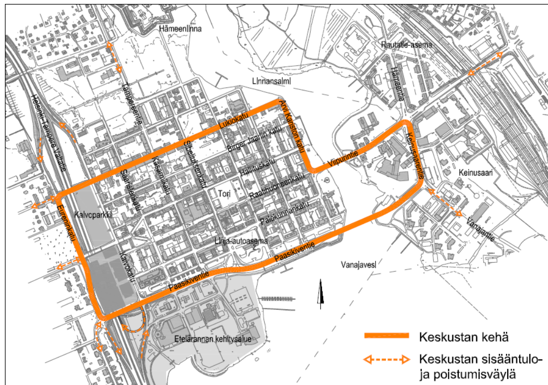
Kuva 9. Keskustan liikenteen kehäratkaisu.
