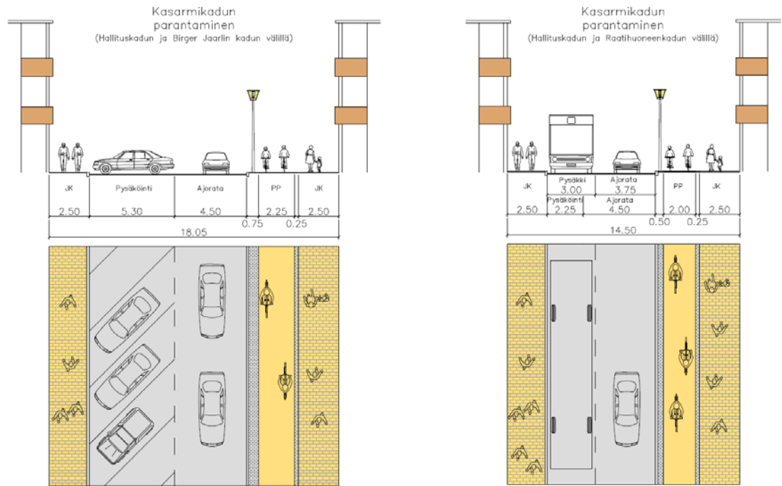
Kuva 18. VE A Kasarmikadun poikkileikkausluonnokset.
