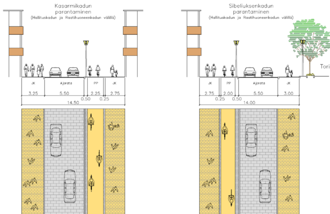
Kuva 21. VE B poikkileikkausluonnokset Kasarmikadulla ja Sibeliuksenkadulla.
