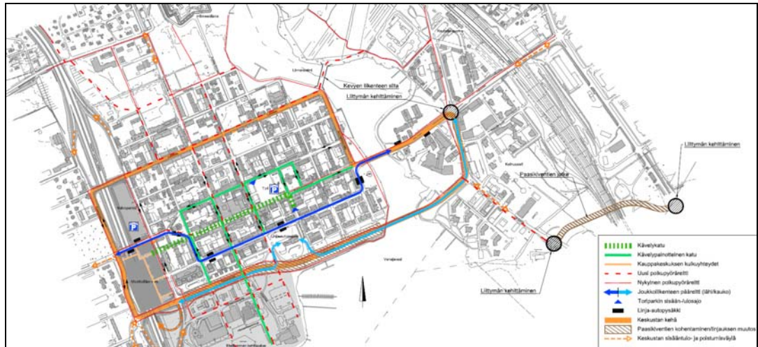
Kuva 20. VE B tavoiteverkko.
