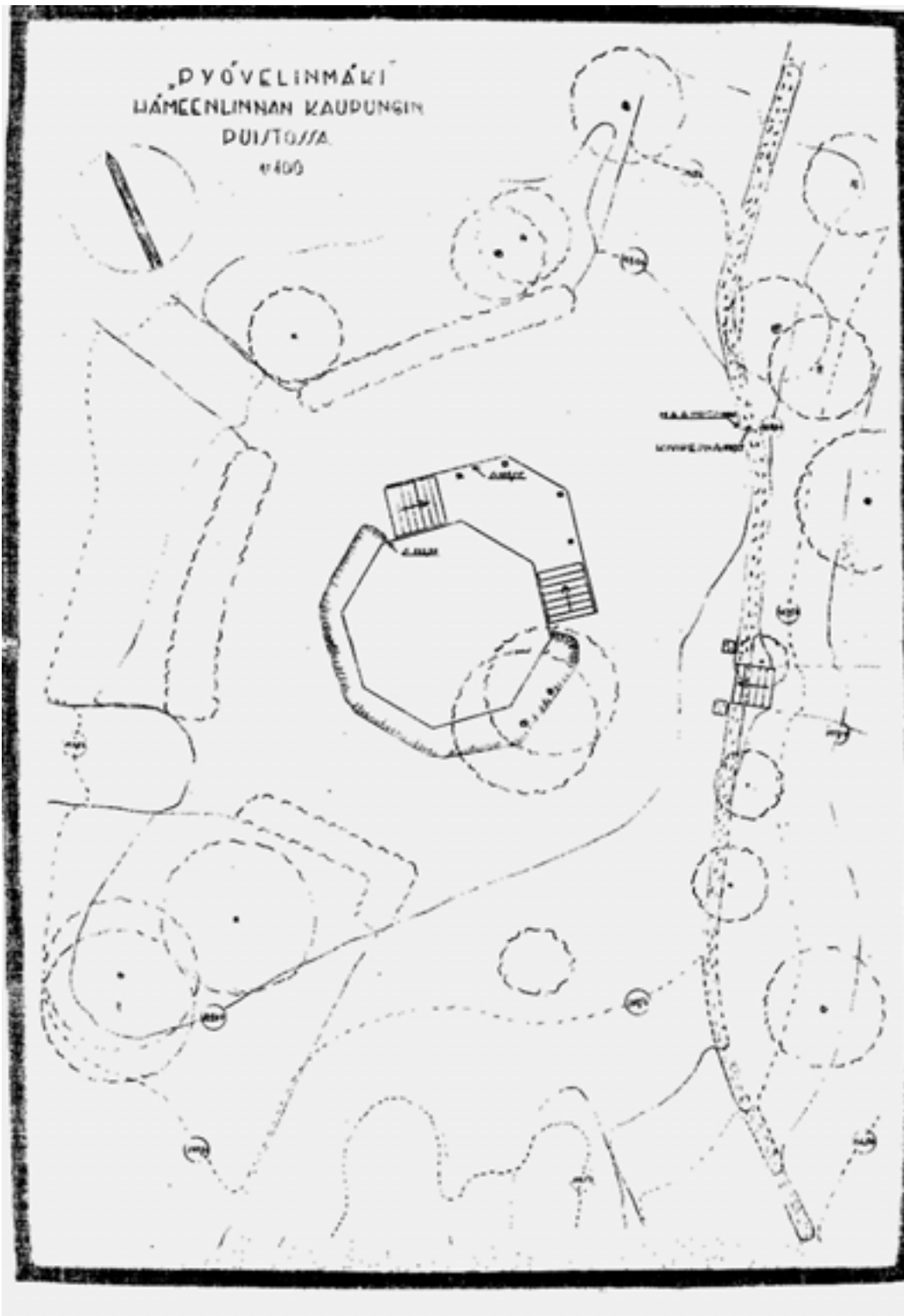
KUVA 43. Puiston korkeimmalla kohdalla sijainneen umpinaisen paviljongin, ns. Kuvernöörin paviljongin, pohjapiirustus. Kukulaa alettiin myöhemmin kutsua aiemmin koko niemeä tarkoittaneella nimellä Pyövelinmäki, siitä piirustuksen otsikko. 1700-luvun puolessa välissä paikka mainitaan nimellä stegelbacken eli teilimäki (Lindeqvist 1926, 368). Itäpuolella näkyy tukimuuri, jolla terassi on pengerretty. Paviljongin kohdalla tukimuurissa on aukko, josta lähtevät portaat ja käytävä alas rinnettä. Paviljongin aukiolta johtaa viisi käytävä eri suuntaan ja sitä ympäröivät toiselta reunalta pensasaidat, ns. syreenimaja. Piirroksessa ei ole päiväystä, mutta arviolta se on 1950-luvulta. (Kuva: TTA).
