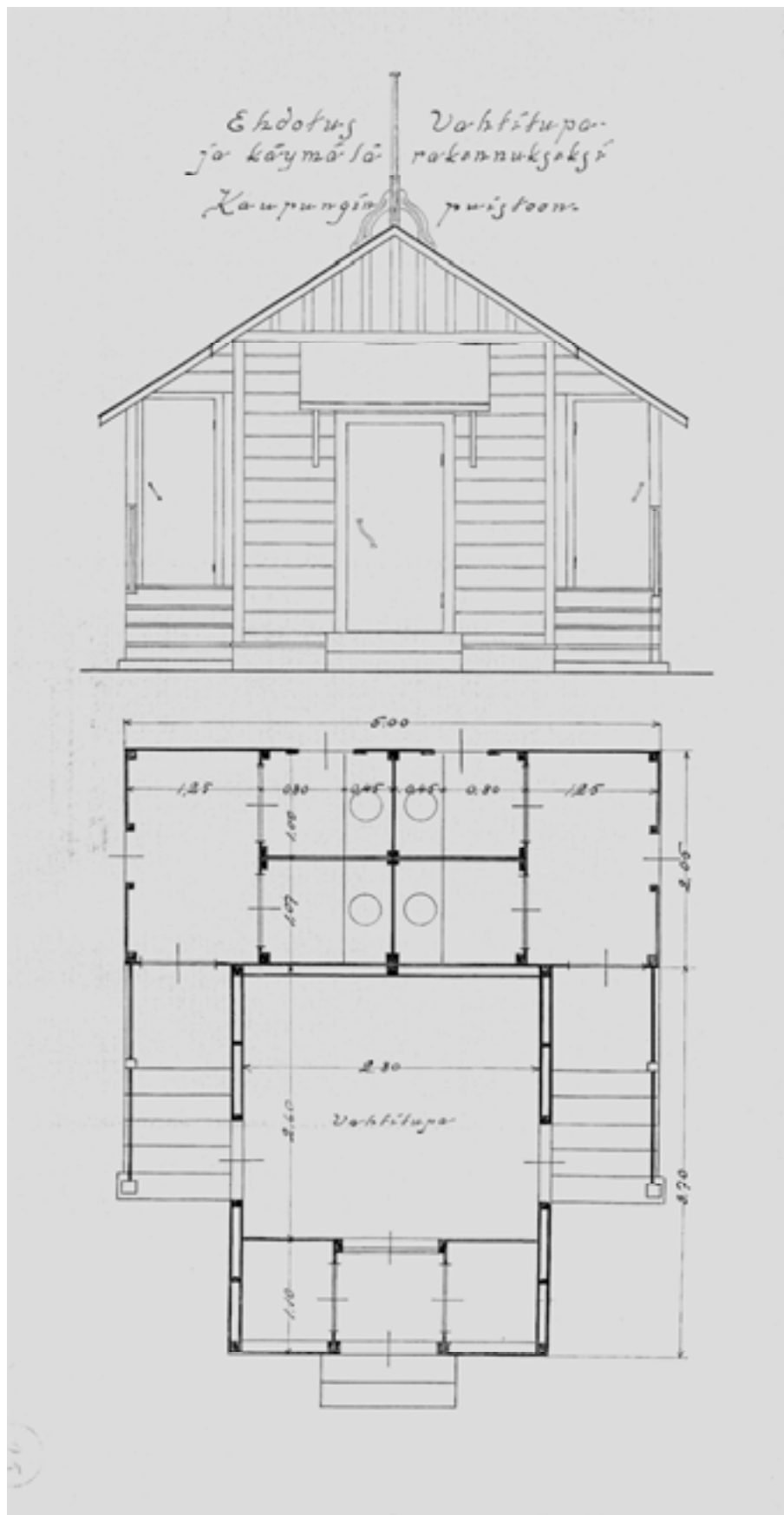
KUVA 80. Päiväämätön ja signeeraamaton piirustus vahtitupa- ja käymälärakennuksesta, joka on saattanut sijaita Parkin pohjoisosassa arviolta vuoden 1937 paikkeilla. (Kuva: TTA).
