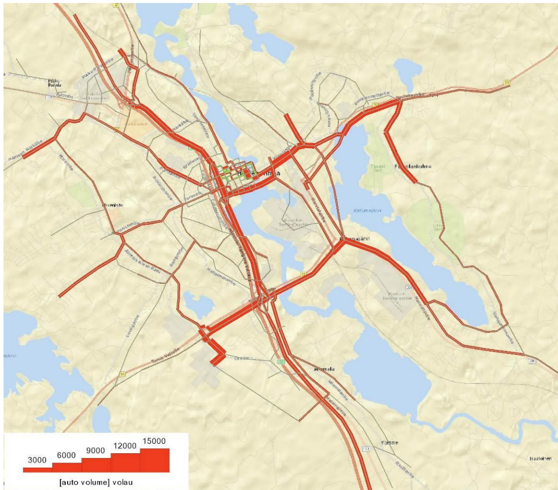
Kuva 4-6: Liikennemäärien muutos ennusteiden 2030+ ja 2030 Malmi välillä nykyverkolla
