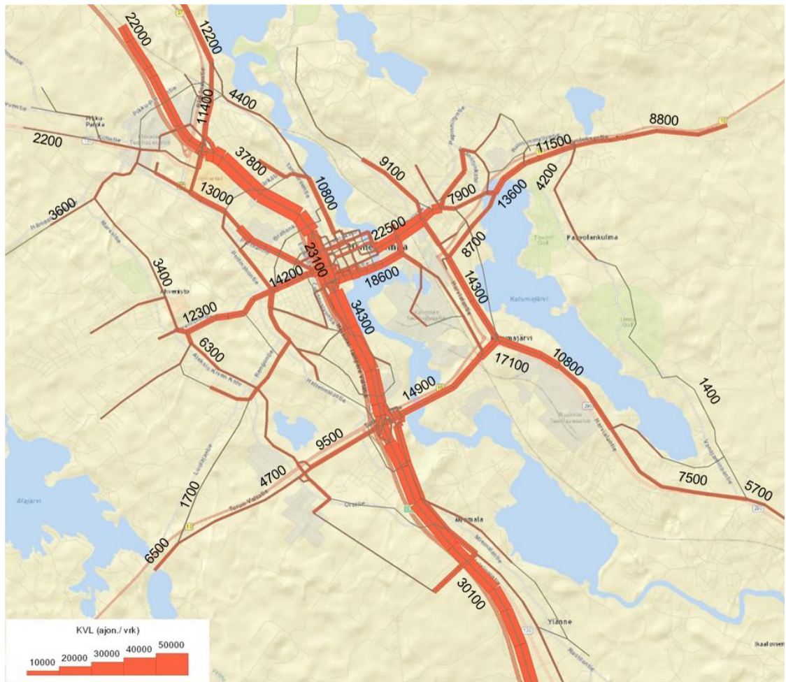
Kuva 4-5: Liikennemäärät ennusteessa 2030 Maltti nykyverkolla
