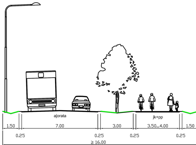
Kuva 3-9 Esimerkki pääkokoojakadun poikkileikkauksesta.
