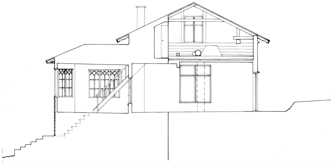
LEIKKAUS A-A 1/50
