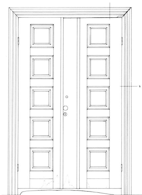
ULKO-OVI 1/10
