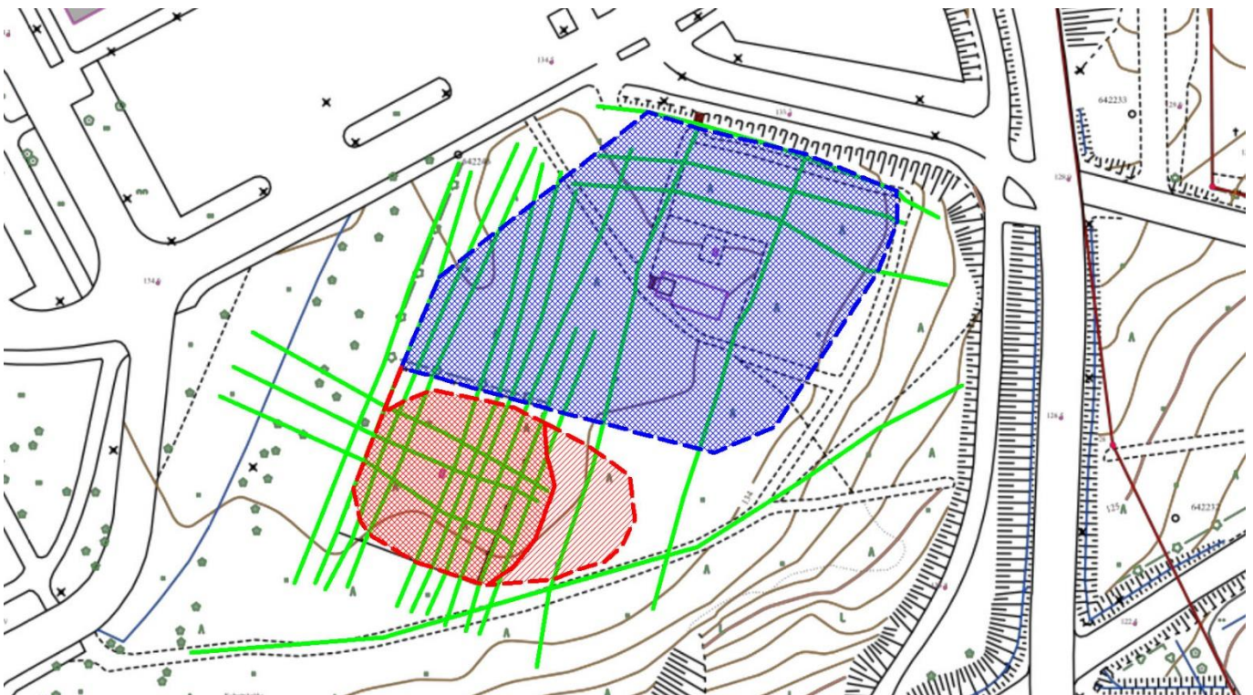
Kartta 10. Maatutkauslinjat ja havaintokohtat. Ei mittakaavassa.
