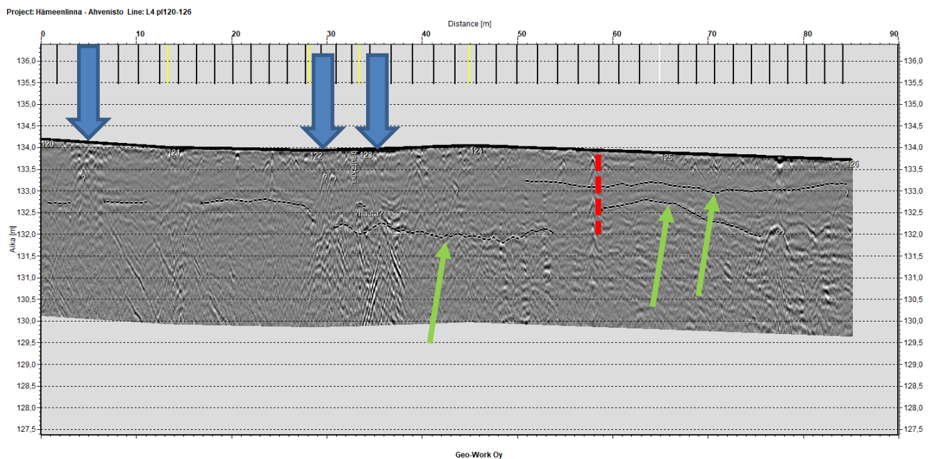
Kuva 8. Maatutkausprofiili (linja 4), jossa erottuu mahdollisia hautoja ja hauta-alueen reuna.
