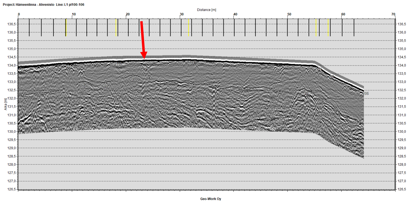
Kuva 7. Linjalla 1 näkyy mahdollisia aidantolpan jäännöksiä (punainen nuoli). Hautauksia tällä hautausmaan koillisreunan linjalla 1 ei voida havaita.
