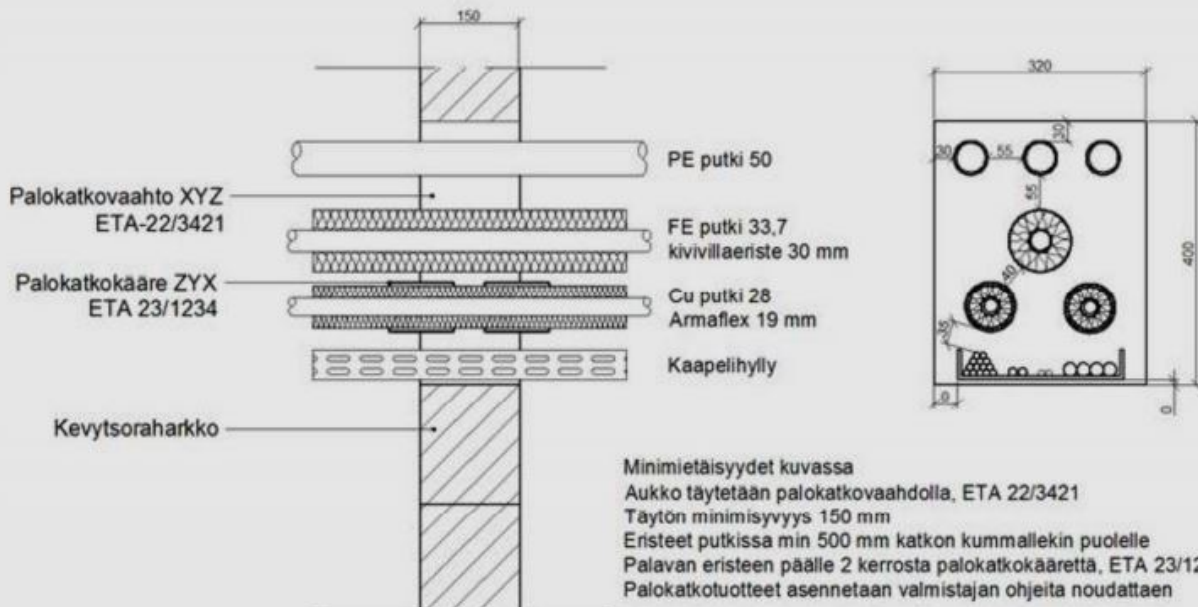
Yhdistelmälapivienti seinässä YS-01, EI60
