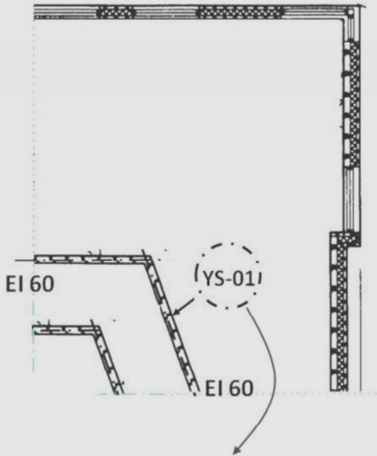
Yhdistelmälapivienti seinässä YS-01, EI60
