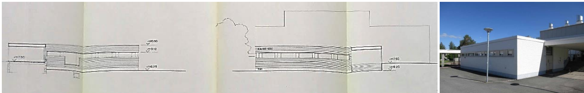
Yllä piirustus: Kirjasto-osan, nykyisen C-osan luoteis- ja koillisjulkisivut 1967, HKA.
