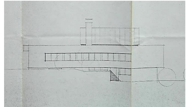
Julkisivut luoteeseen ja kaakkoon, Unto Ojonen 1963, HKA.
