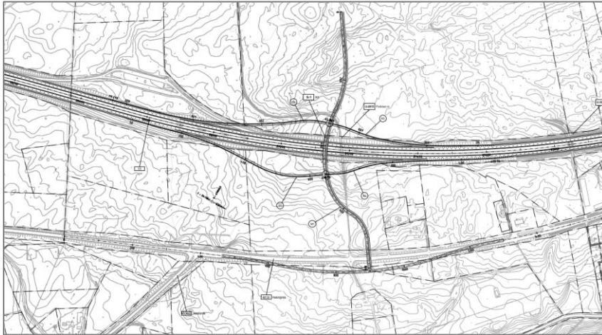
Kuva 3-1. Eritasoliittymävaihtoehto A.
