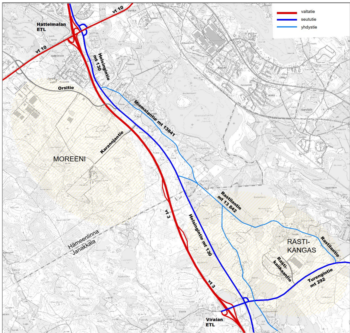
Kuva 2-3. Suunnittelualan tieverkko.
