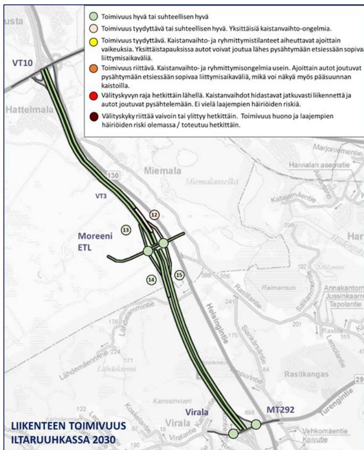
Kuva 16. Liikenteen toimivuus Vt3:lla iltaruuhkatunnin aikana 2030, kun Moreenin ETL on toteutettu.
