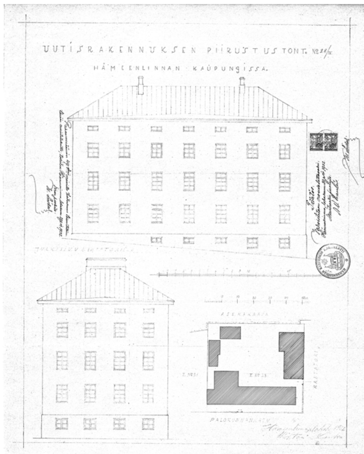
YLLÄ VASEMALLA/ Arjanlinnan "uutisrakennuksen" suunnitelma vuodelta 1932. 1
