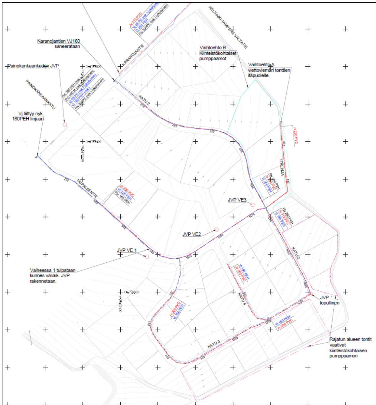
Kuva 20. Vesihuollon yleissuunnitelma. Kuvan lounaiskulman linjasta on luovuttu, koska tonttijako alueella ei ole kuvan mukainen.
