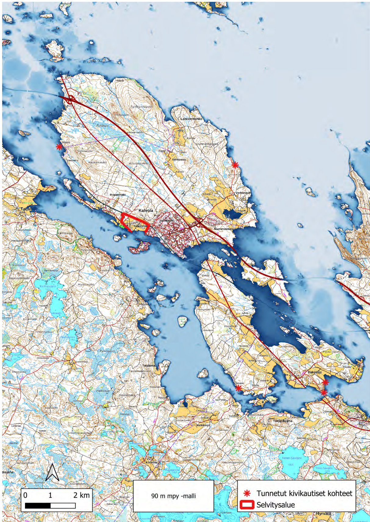
Kuva 3. Muinaisranta-malli, jossa merenpinta nostettu tasolle 90 m mpy. Tällöin alue on ollut osa Ancyclusjärveä. Kartan piirtänyt Mikko Ahvonen.
