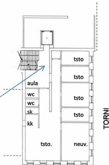
Tornin 4. kerros
