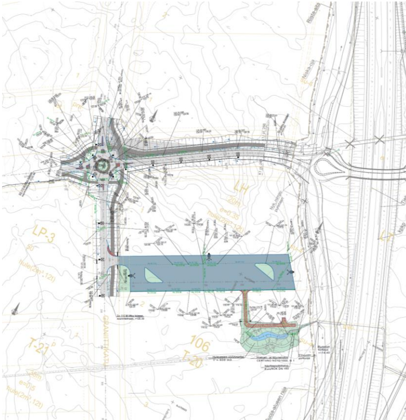
Kuva 25. Kuivatussuunnitelma.
