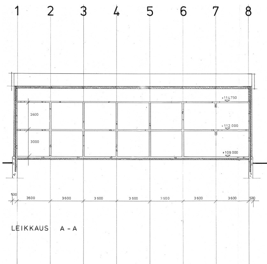
Kuva 74: Leikkaukset - Oppilasasuntola 3, 1975
