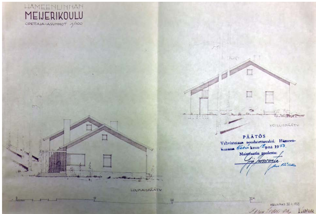
Kuva 55: Julkisivut lounaaseen ja koilliseen - Opettaja-asunnot, 1954
