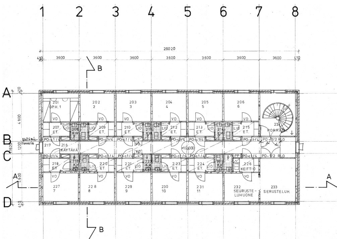
Kuva 70: Pohjapiirustus - 2. Kerros, oppilasasuntola 3, 1975
