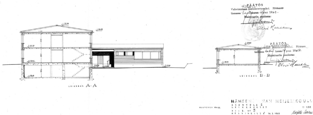
Kuva 67: Leikkaukset - Oppilasasuntola 2, 1964
