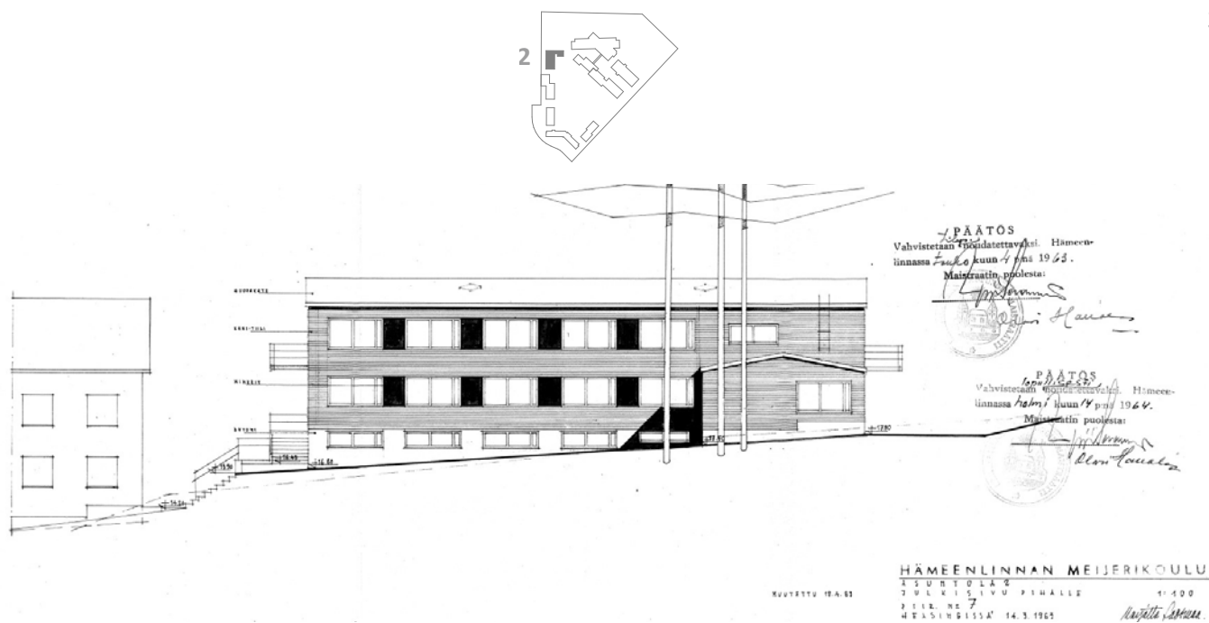
Kuva 65: Julkisivu itään - Oppilasasuntola 2, 1964
