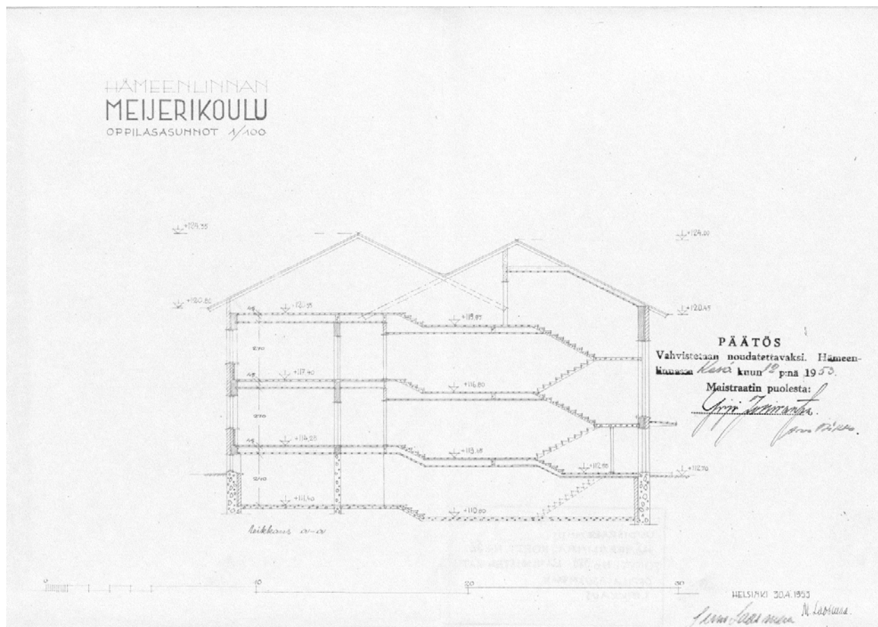
Kuva 49: Leikkaus - Oppilasasuntola 1, 1954
