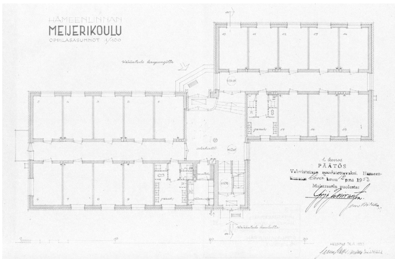
Kuva 42: Pohjapiirustus - 1. Kerros, Oppilasasuntola 1, 1954
