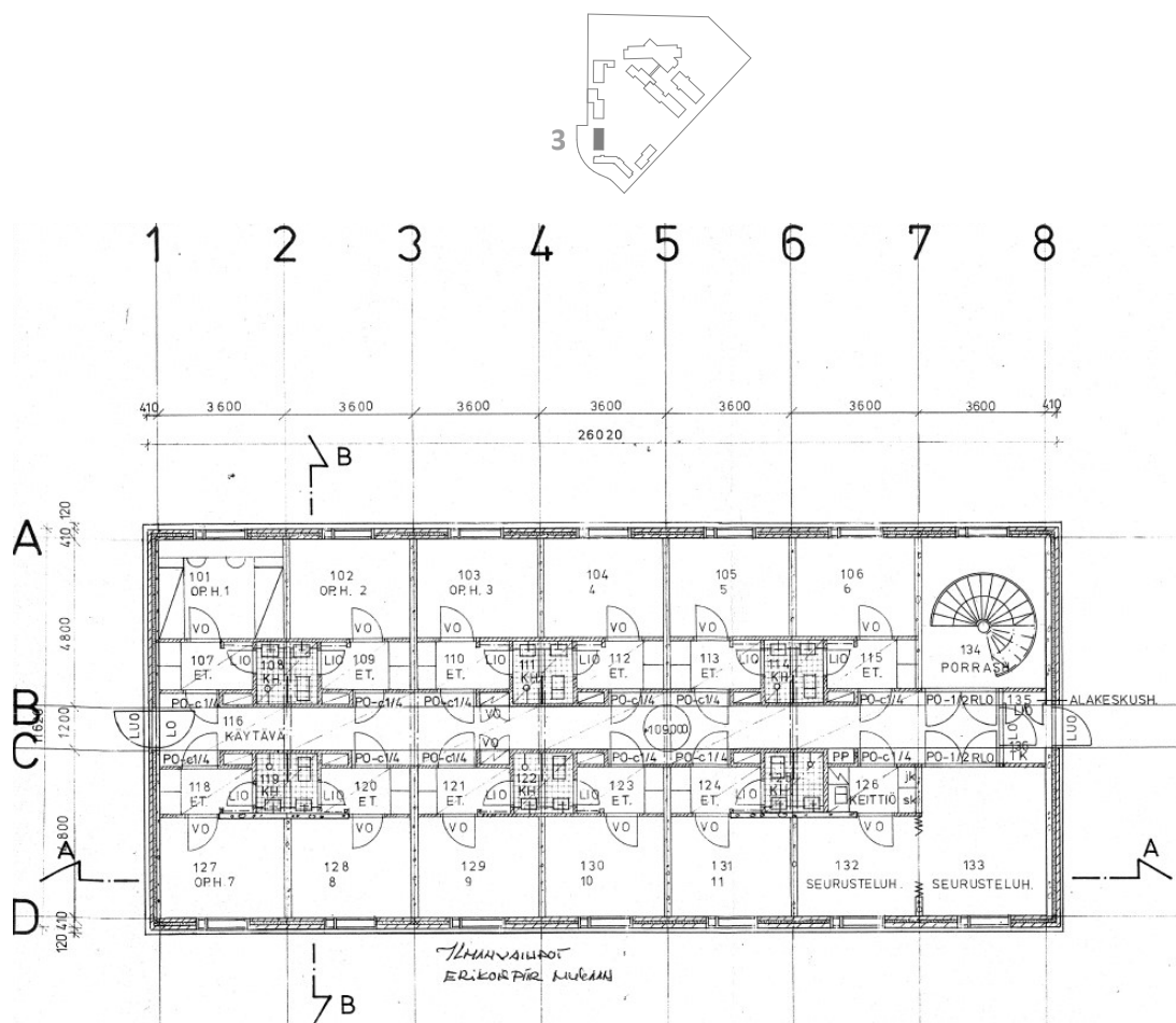
Kuva 69: Pohjapiirustus - 1. Kerros, oppilasasuntola 3, 1975
