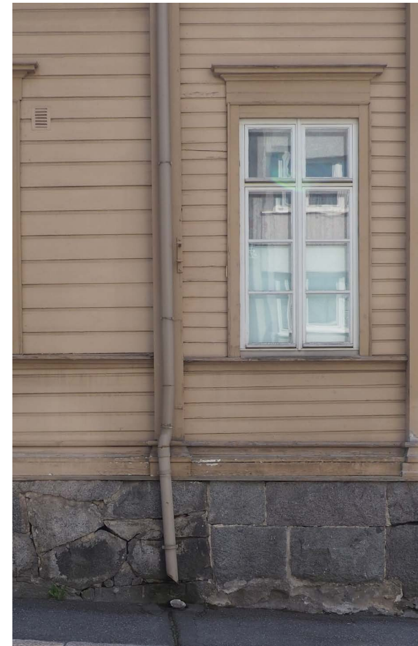
Pohjoisjulkisivun julkisivulaudoituksen leveydestä ja sokkelikivien muodosta on erotettavissa kohta, jossa vuoden 1858 rakennusosa vaihtuu uudempaan. Kapea pilasterien väli on osin 1930-luvulta, jolloin kadunpuoleinen sisäänkäynti poistettiin. Sen oikealla puolella sokkeli ja julkisivun puuosat ovat vuodelta 1895.
