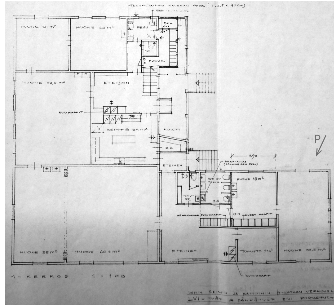
1. kerroksen pohjapiirros 1970-luvulta. (Kuva: Hämeenlinnan kaupunginarkisto)
