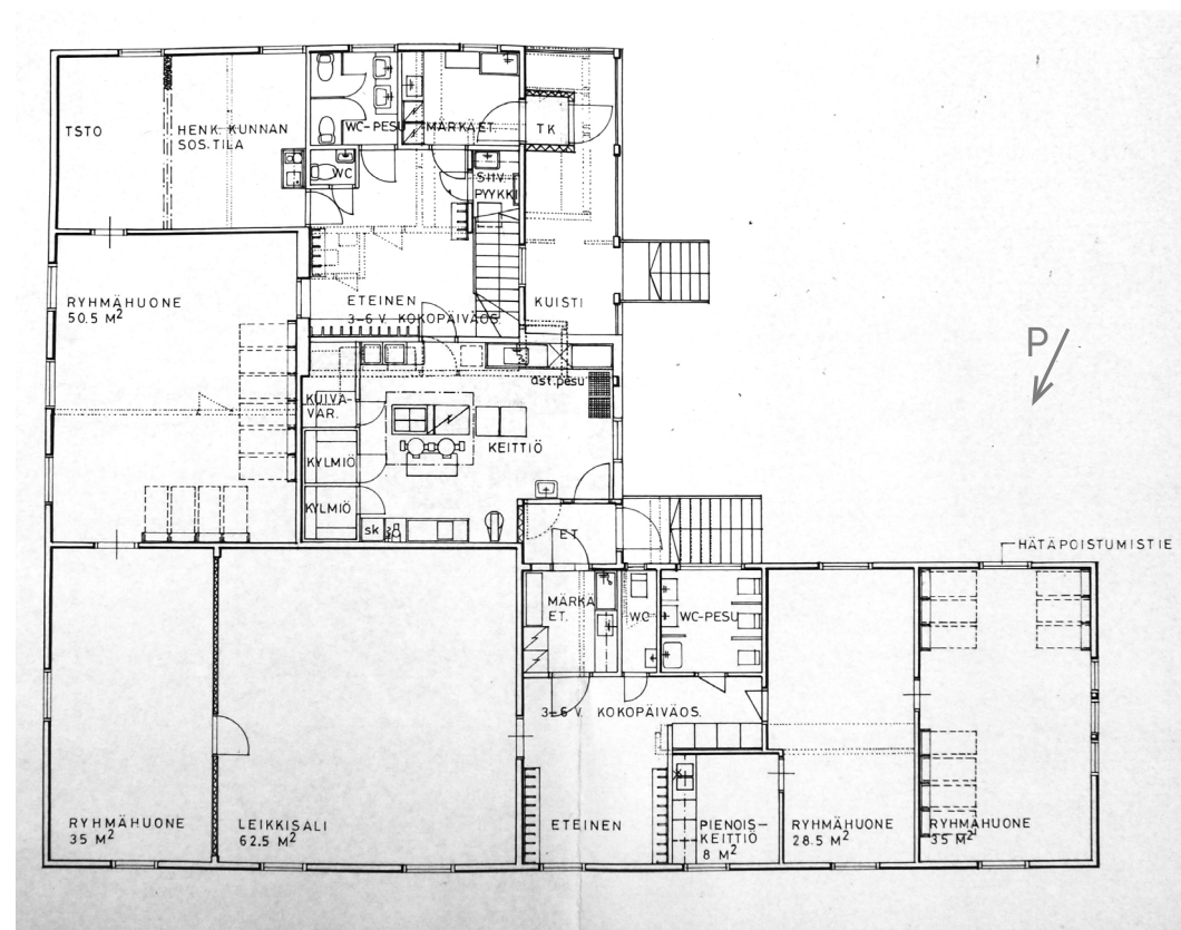
1. kerroksen pohjapiirros 1980-luvulta. Suurin osa kuvassa esitetyistä muutoksista jätettiin toteuttamatta. (Kuva: Hämeenlinnan kaupunginarkisto)
