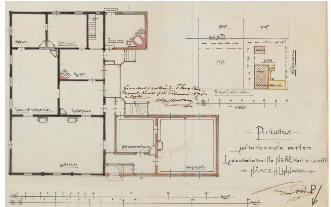
Vuoden 1895 laajennussuunnitelma, jonka on laatinut arkkitehti Henrik R. Helin. Pohja- ja asemapiirros on esitetty siten, että pohjoinen on kuvissa alhaalla. (Kuva: Kansallisarkisto)
