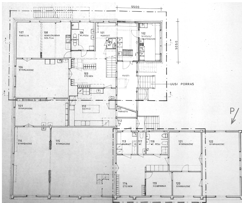
1. kerroksen muutospiirros vuodelta 1995. (Kuva: Hämeenlinnan kaupunginarkisto)
