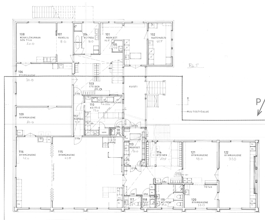
1. kerroksen muutospiirros vuodelta 1997. (Kuva: Hämeenlinnan kaupunki, Tilapalvelut)
