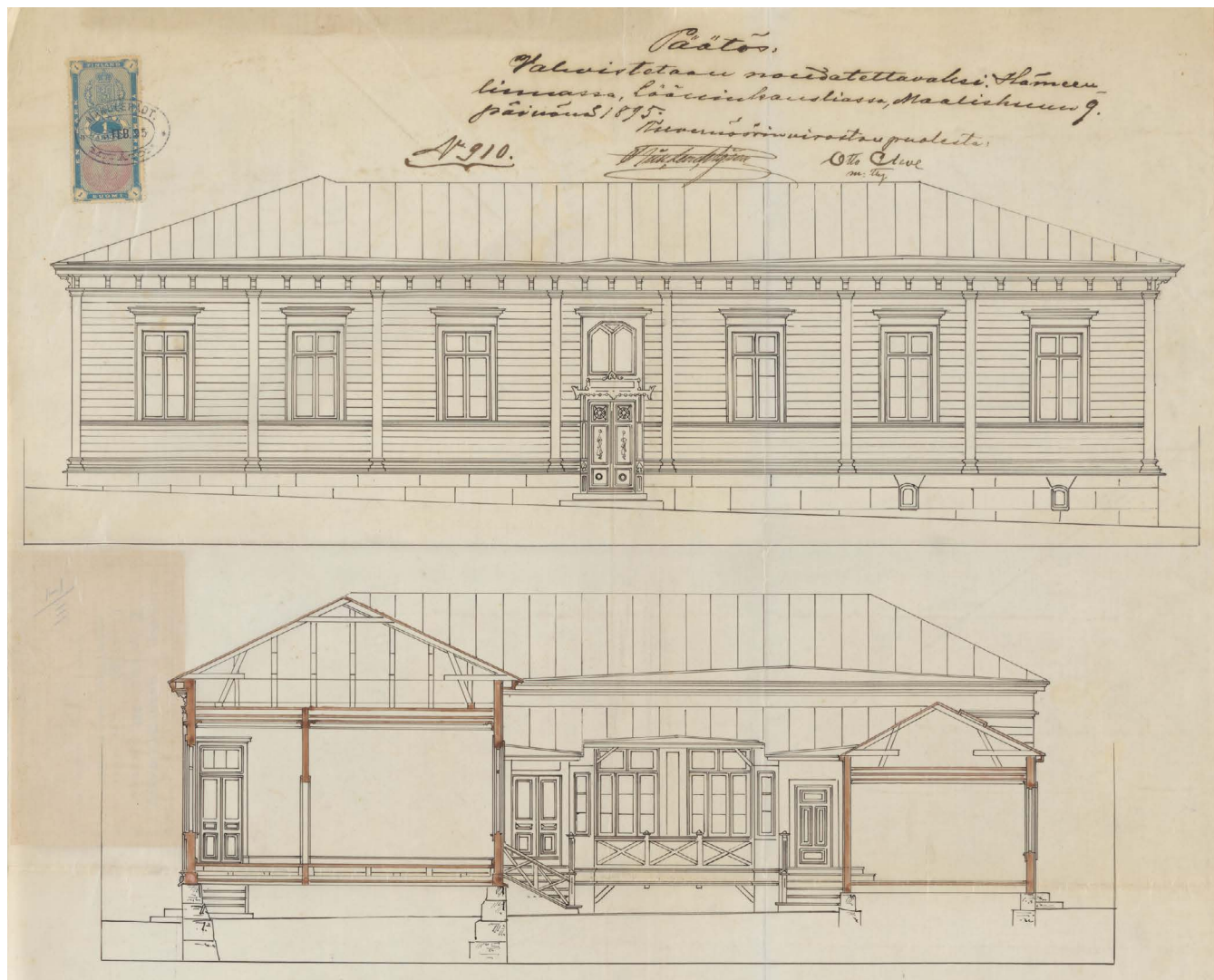
Vuoden 1895 laajennussuunnitelma, jonka on laatinut arkkitehti Henrik R. Helin. (Kuva: Kansallisarkisto)
