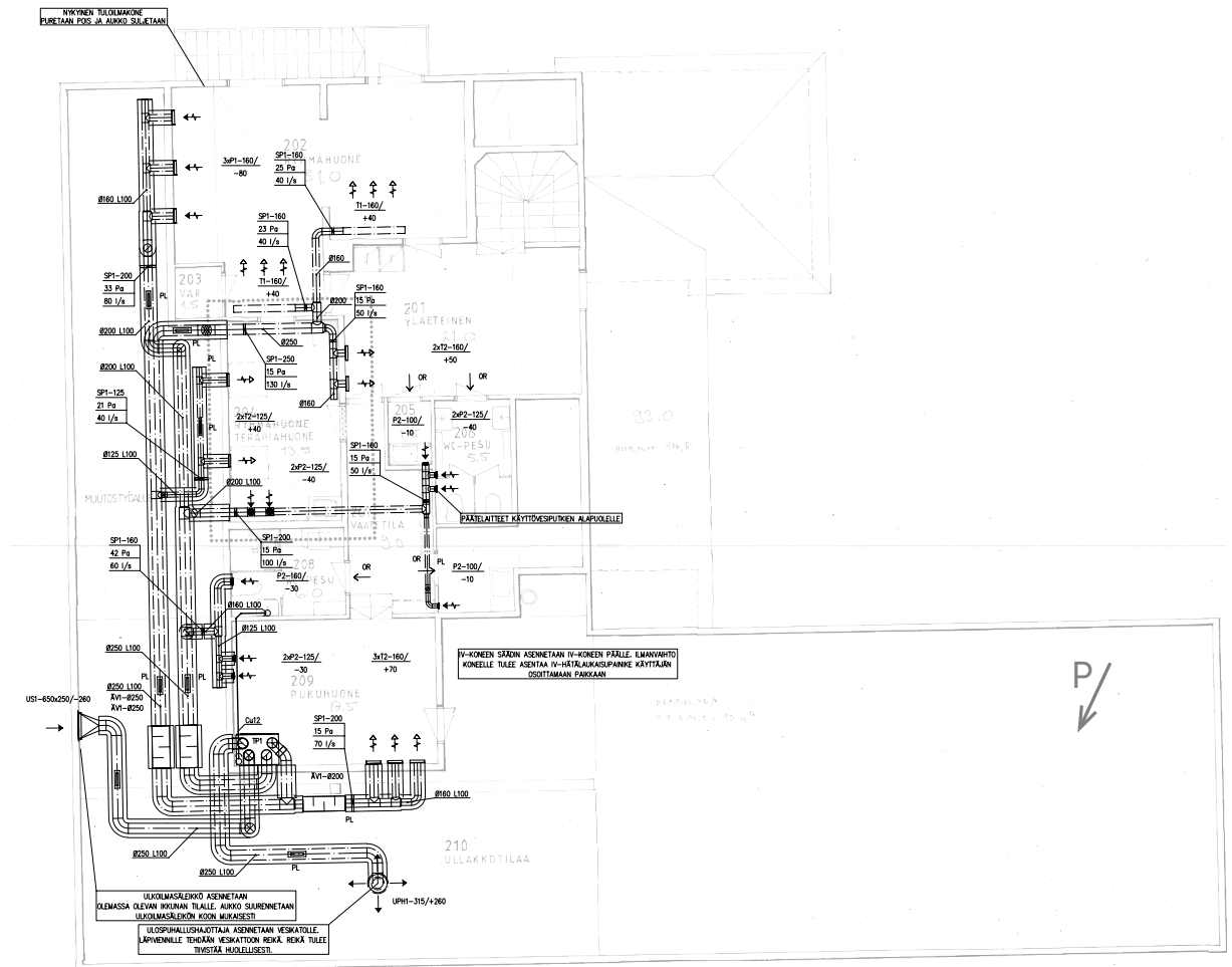
Ilmanvaihtopiirros vuodelta 2021. (Kuva: Hämeenlinnan kaupunki, Tilapalvelut)
