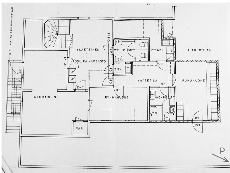
2. kerroksen pohjapiirros 1980-luvun muutoksista. (Kuva: Hämeenlinnan kaupunginarkisto)
